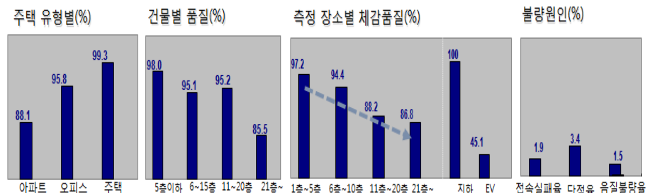
(그림 10) 고층의 공동주택에서의 전파음영 현장측정 결과
