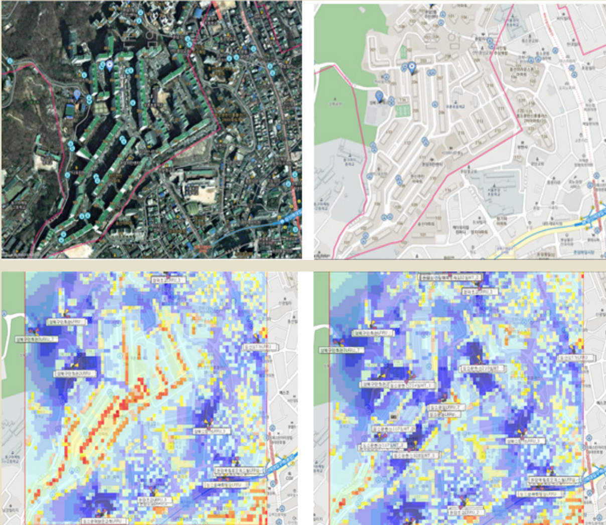
단지 내 시설 전 RSRP
